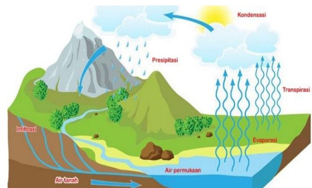
Gambar 1. Siklus Hidrologi (sumber :google)
